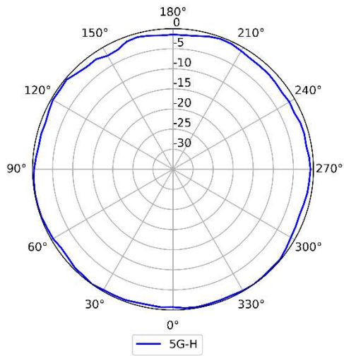
5GHz (Horizontal)
